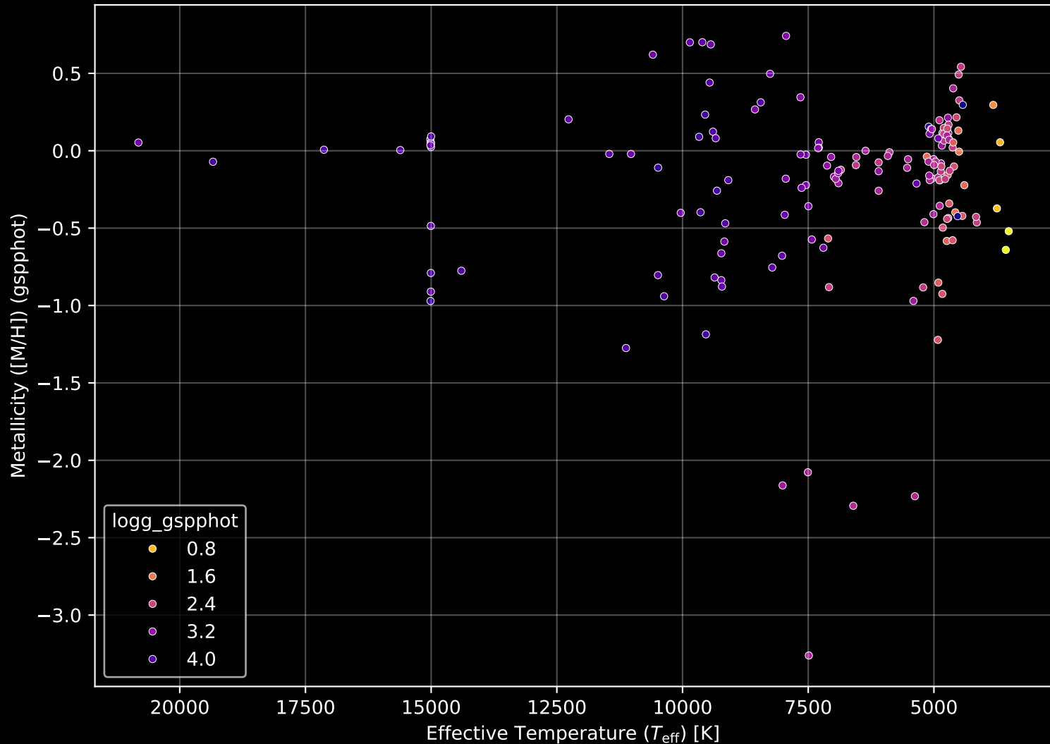
APOGEE DR17 Field: [083+04] Stellar Population Parameters (n= 161)
